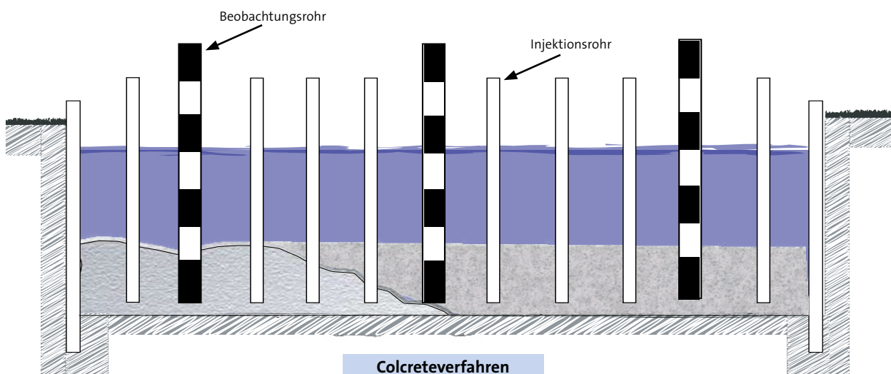
Abb. 8.12.11 Colcreteverfahren
