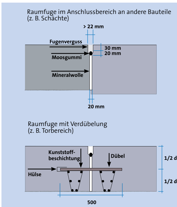
Abb. 8.4.26 Bewegungsfuge/ Raumfuge
