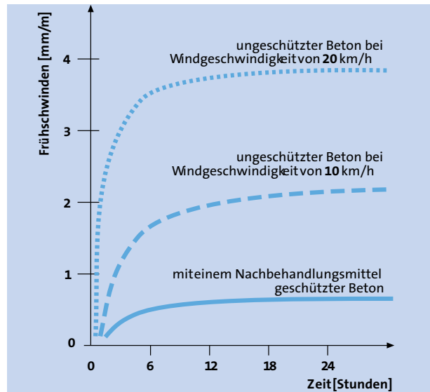
Abb. 5.2.4 (links) Einfluss des Feuchthaltens auf die Festigkeitsentwicklung des Betons im Oberflächenbereich
