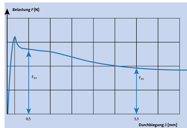
Abb. 8.16.5 Lastdurchbiegungsbeziehung zur Ermittlung der Nachrissbiegezugfestigkeiten
