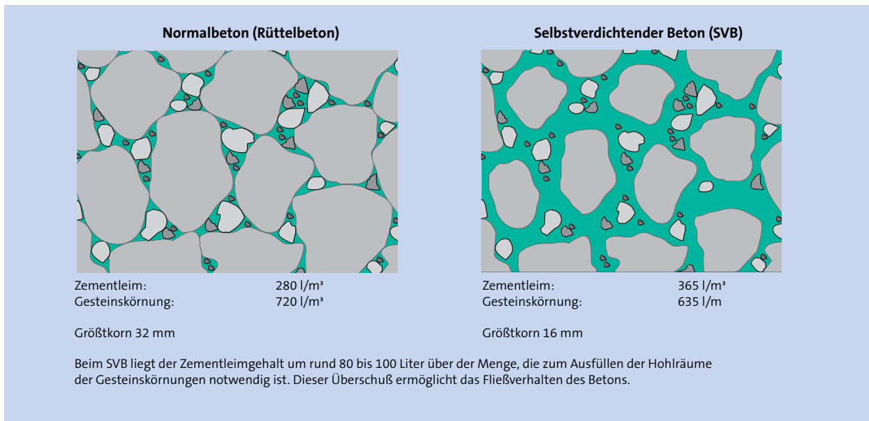
Abb. 7.5.5 Unterschiedliche Volumenverhältnisse von Normalbeton und selbstverdichtendem Beton
