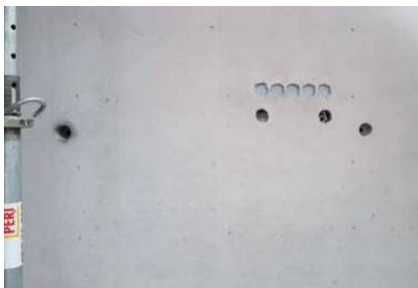
Abb. 7.15.5 R-Beton - Detailaufnahme Sichtbeton
