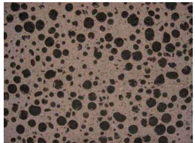
Abb. 7.6.12 Leichtbeton mit Blähton als grobe Gesteinskörnung - Oberfläche geschliffen
