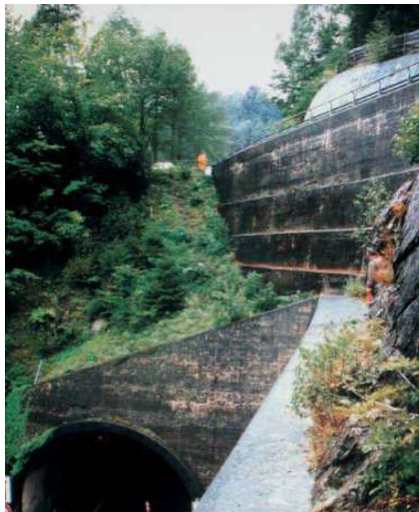
Abb. 10.7.16 Starke AKR-Schäden an einem Tunnelgewölbe
