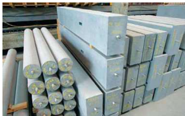
Abb. 7.5.3 Hochwertige Fertigteile aus SVB
