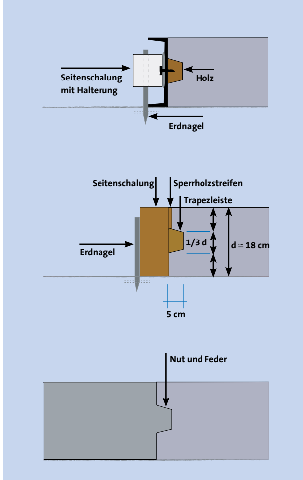
Abb. 8.4.23 Pressfuge/Arbeitsfuge Variante 1
