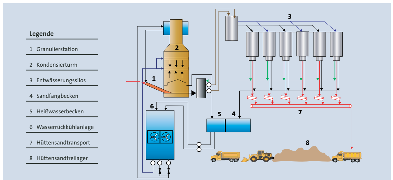
Abb. 1.1.10 Hüttensand
