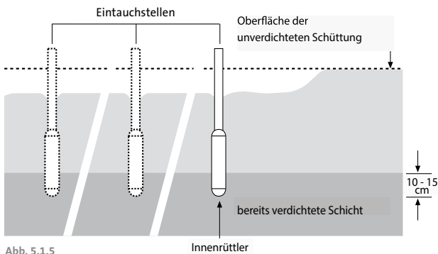
Abb. 5.1.5 Frischbetoneinbau und Verdichtung
