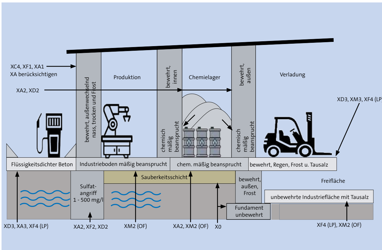
Abb. 3.3.7 Expositionsklassen am Beispiel einer Prinzipskizze für den Industriebau
