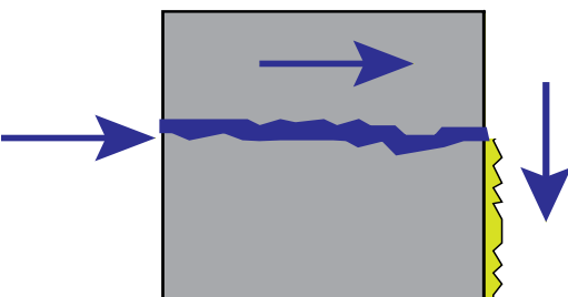
Abb. 10.2.3 Kalkaussinterungen/ Kalkauswaschungen
