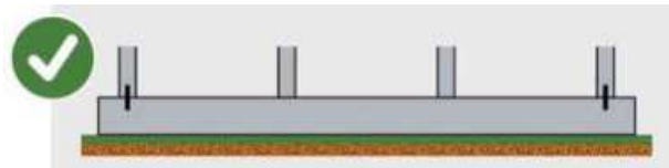
Abb. 8.13.3 Gleitlagerung - geringer Grad an Behinderung
