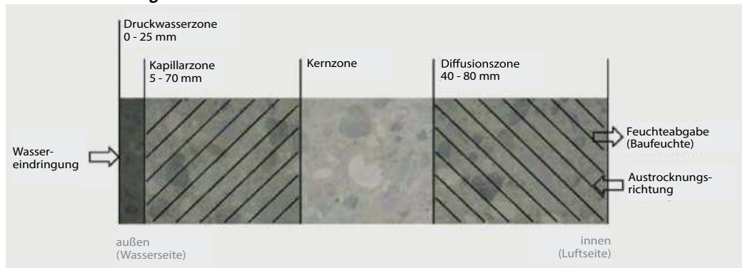
Abb. 8.13.1 WU-Beton mit 240 mm Wandstärke
