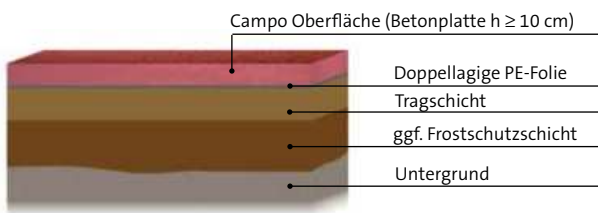
Abb. 7.11.6 Aufbau CampoDrain
