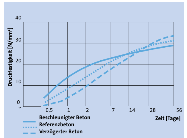
Abb. 1.5.6 Wirkung von Verzögerer und Beschleuniger auf die Betonfestigkeit
