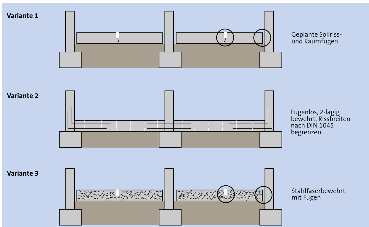
Abb. 8.4.31 Konstruktion beeinflusst Fugenplanung
