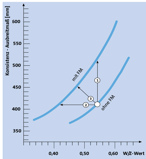
Abb. 1.5.3 Auswirkungen von Fließmitteln
