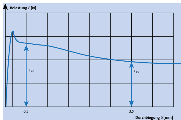
Abb. 7.8.4 Last-Durchbiegungs-Beziehung zur Ermittlung der Nachrissbiegezugfestigkeiten
