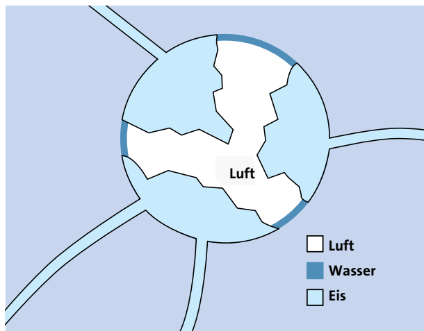
Abb. 1.5.5 Eisbildung in der Luftpore (schematisch)
