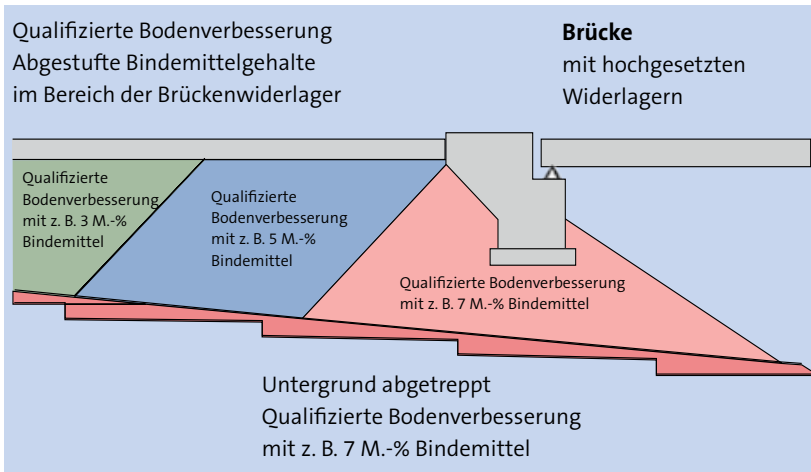
Abb. 8.18.1 Qualifizierte Bodenverbesserungen
