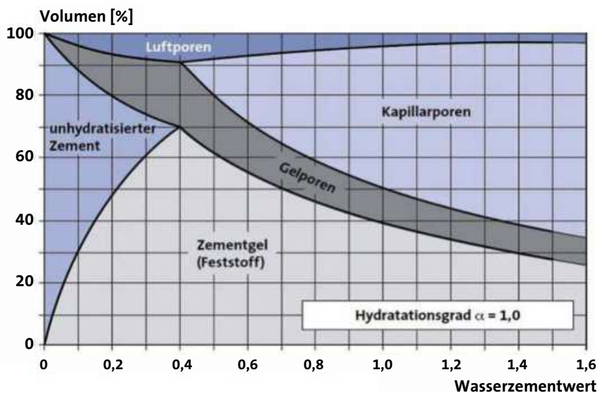
Abb. 3.1.3 Zusammensetzung des Zementsteins in Abhängigkeit des Wasserzementwertes
