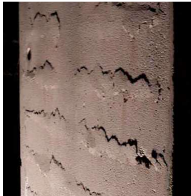
Abb. 10.8.4 Schäden an der Betonoberfläche durch Karbonatisierung
