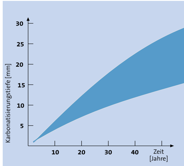
Abb. 10.8.3 Die Karbonatisierungstiefe als Funktion der Zeit variiert - je nach den einwirkenden Faktoren - in einem weiten Bereich
