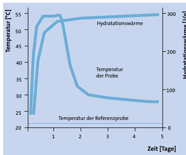
Abb. 1.1.31 Verlauf von Temperatur und Hydratationswärme eines CEM I 42,5 N im Versuch nach Langavant
