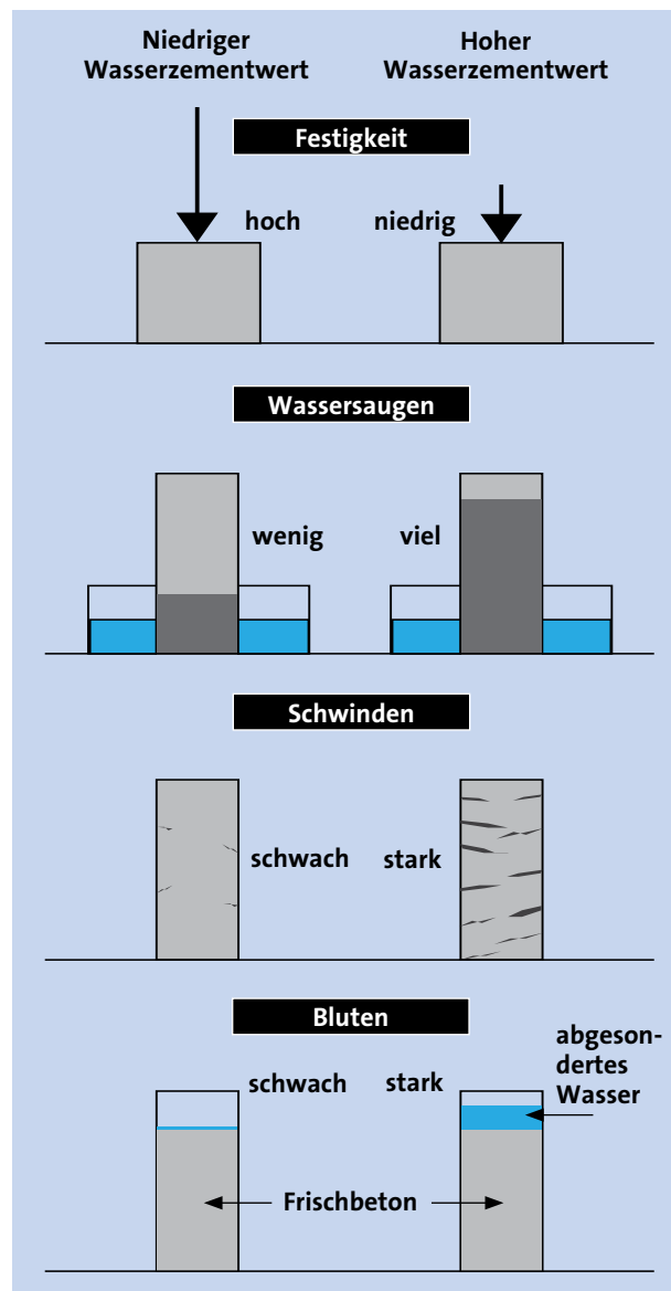
Abb. 3.1.6 Einfluss des Wasserzementwertes auf Betoneigenschaften
