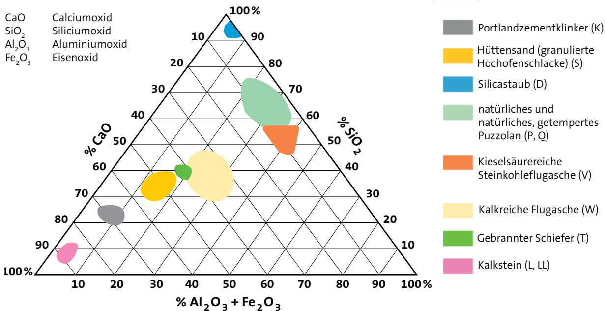
Abb. 1.1.25 Dreistoffdiagramm
