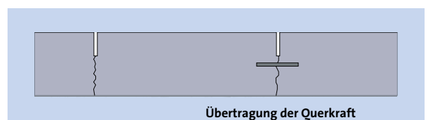
Abb. 8.4.18 Verdübelung der Scheinfuge
