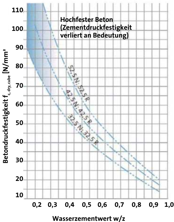
Abb. 3.1.5 Walz-Diagramm
