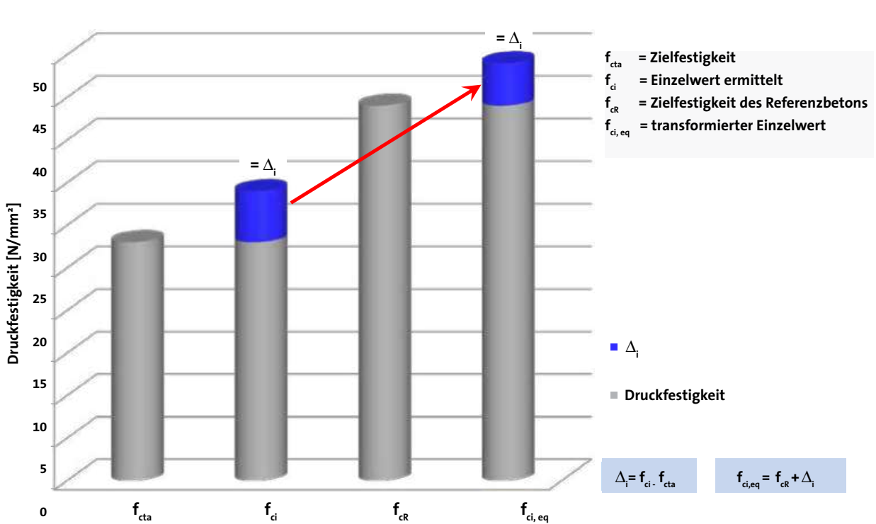
Abb. 6.1.10 Funktion und Darstellung des Differenzverfahrens
