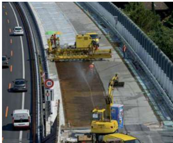
Abb. 7.13.4 Anwendung bei Brückensanierung
