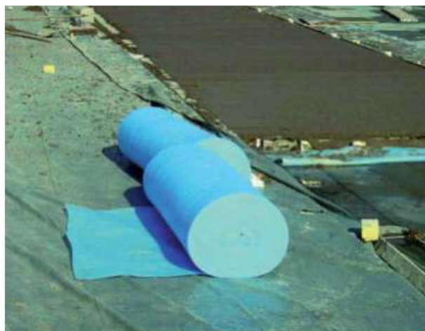
Abb. 8.5.4 Bereithalten wärmedämmender Nachbehandlungsmatten
