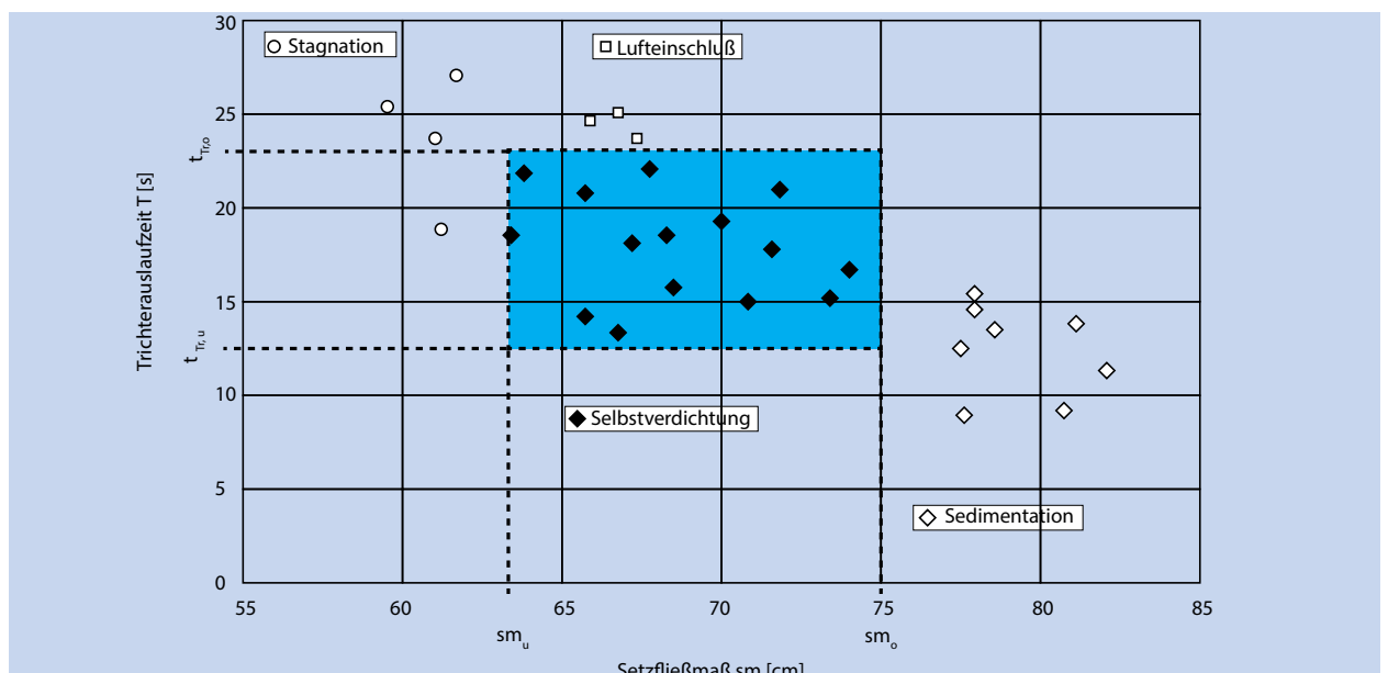
Abb. 7.5.11 Beispiel für einen Verarbeitbarkeitsbereich eines selbstverdichtenden Betons
