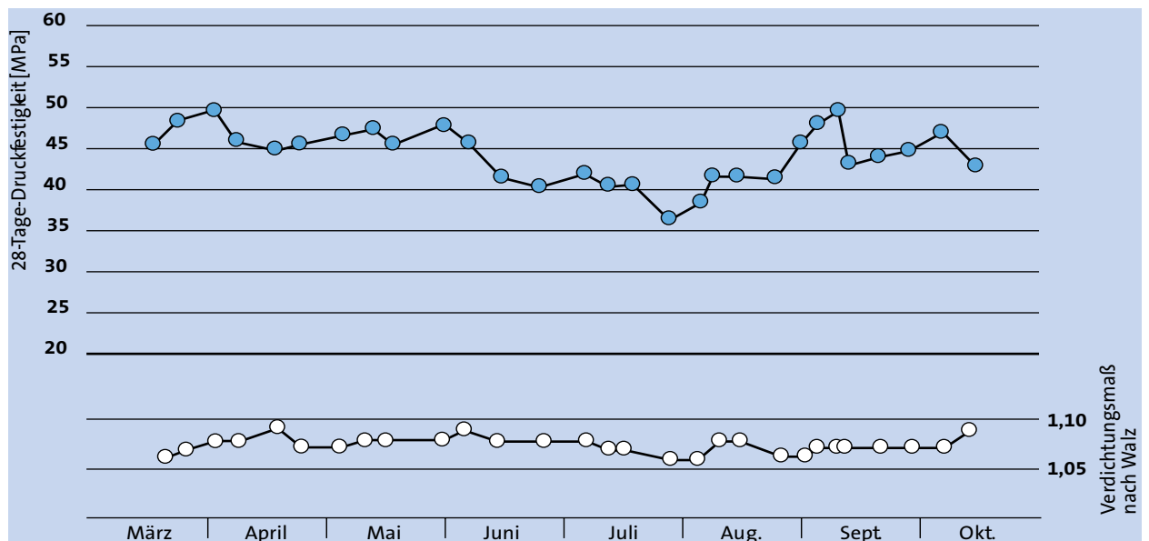
Abb. 5.3.1 Typische Betonfestigkeitsstatistik während des Sommerhalbjahrs. Daten aus der Qualitätssicherung eines Transportbetonwerks
