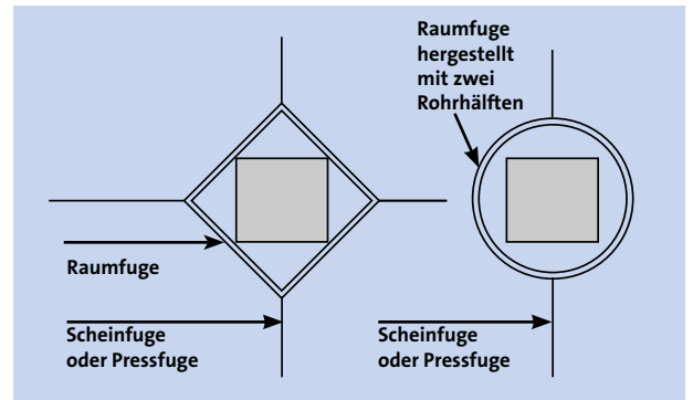
Abb. 8.4.36 Vorschläge der Fugenanordnung bei Stützen, Schächten und Einbauteilen
