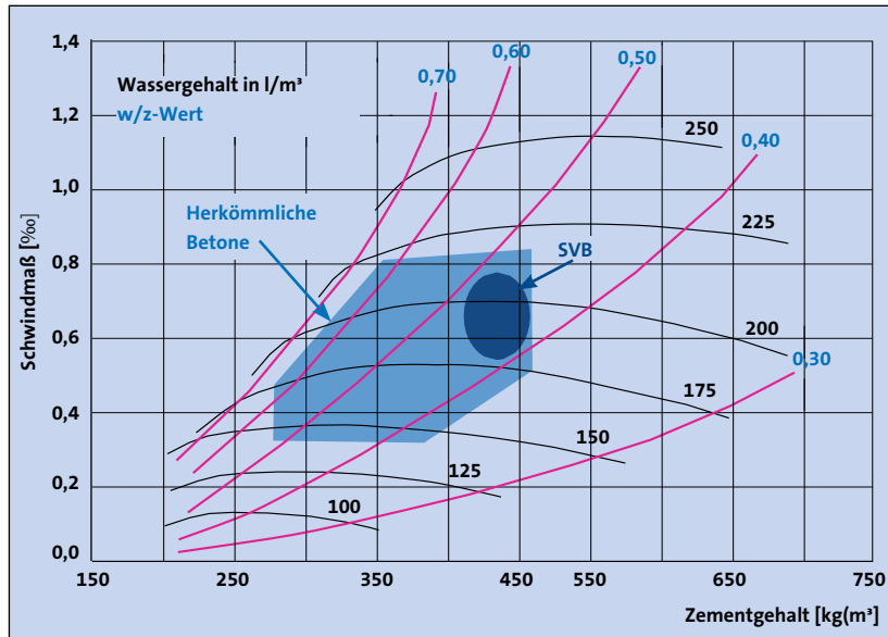
Abb. 10.3.11 Einfluss des Zementgehalts, des Wassergehalts und des Wasserzementwerts auf das Endschwindmaß (gemessen an Prismen der Abmessungen 100 x 100 x 400 mm 3 bei einer relativen Luftfeuchte von 50 % ab dem fünften Tag) (Quelle: P. Grübl, H. Weigler, S. Karl: Beton-Arten, Herstellung und Eigenschaften, Verlag Ernst & Sohn)
