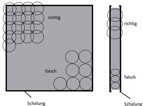
Abb. 5.1.7 Überschneiden der Wirkungsbereiche (links); Abstimmen der Größe der Vibriernadel auf die Bauteilabmessungen (rechts)
