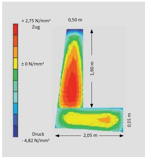
Abb. 10.3.9 Betonspannungen infolge Hydratationswärme in einer dicken Stützmauer. Skala der berechneten Spannungen links und Maßangaben rechts
