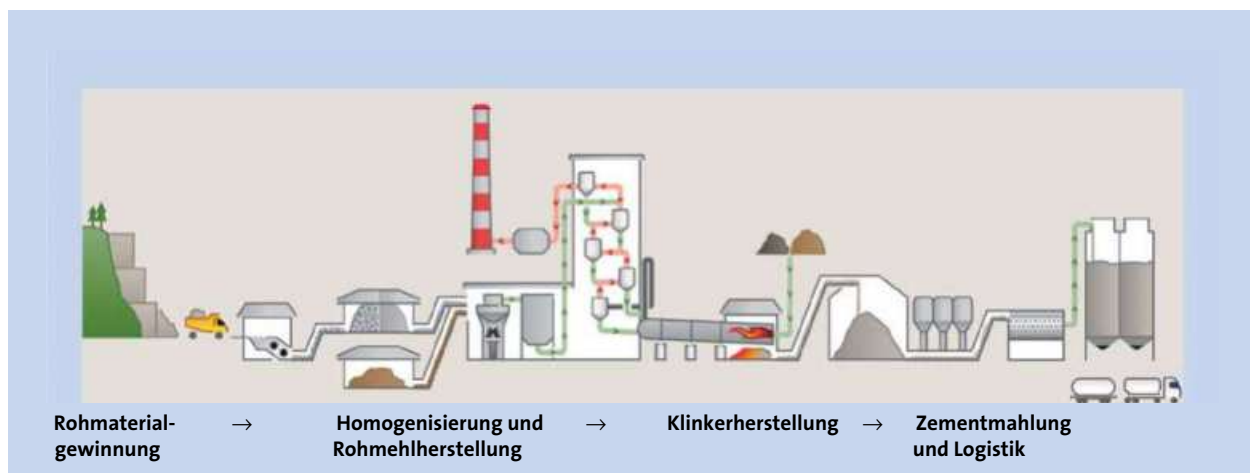
Abb. 1.1.8 Produktionsschema Zementherstellung
