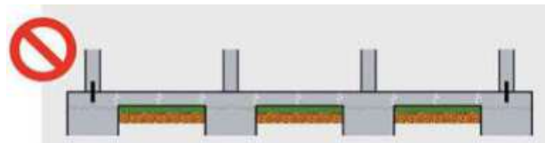
Abb. 8.13.4 Voller Zwang der Sohlplatte
