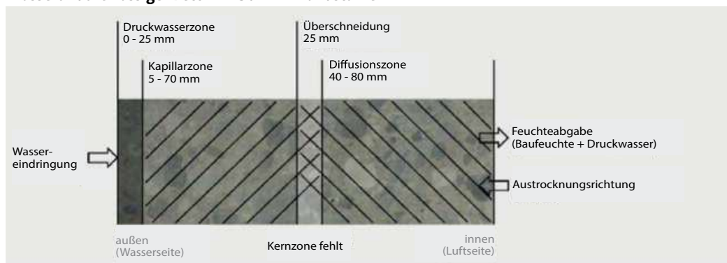
Abb. 8.13.2 WU-Beton mit 150 mm Wandstärke
