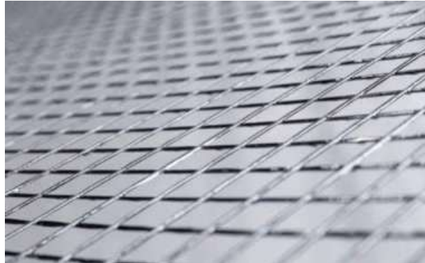
Abb. 9.5.7 solidian GRID Bewehrungsgitter aus Carbon, das mit innovativer und zukunftsweisender Technologie hergestellt wird Bild: solidian GmbH
