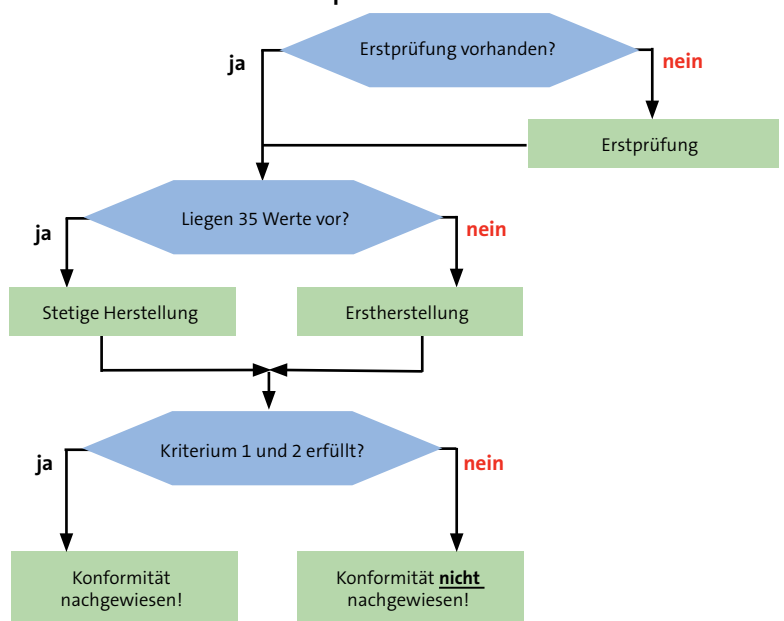
Abb. 6.1.7 Flussdiagramm für die Konformitätskontrolle im Transportbetonwerk
