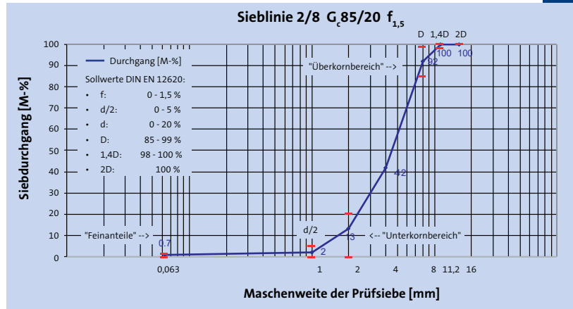
Abb. 1.3.9 Korngemischabstufung in der Sieblinie
