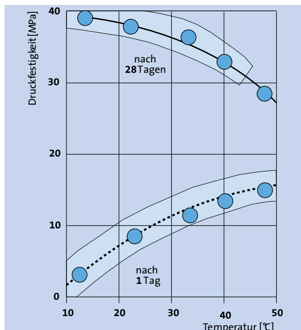
Abb. 5.3.2 Auswirkung der Temperatur auf die Entwicklung der Druckfestigkeit von Beton
