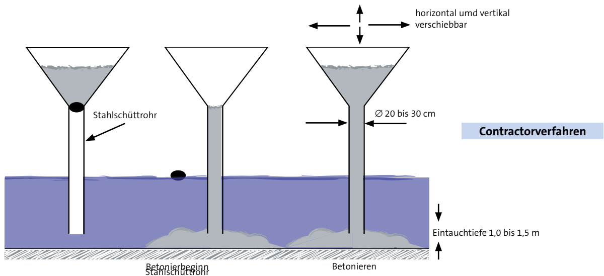
Abb. 8.12.8 Contractorverfahren
