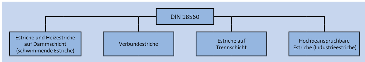
Abb. 7.12.3 Einteilung der Estriche nach nationaler Normung
