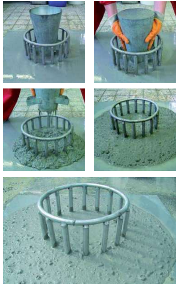
Abb. 7.5.6 bis 7.5.10 Messung des Setzfließmaßes mit Blockiererring sm , sowie Fließzeit t_{500}
