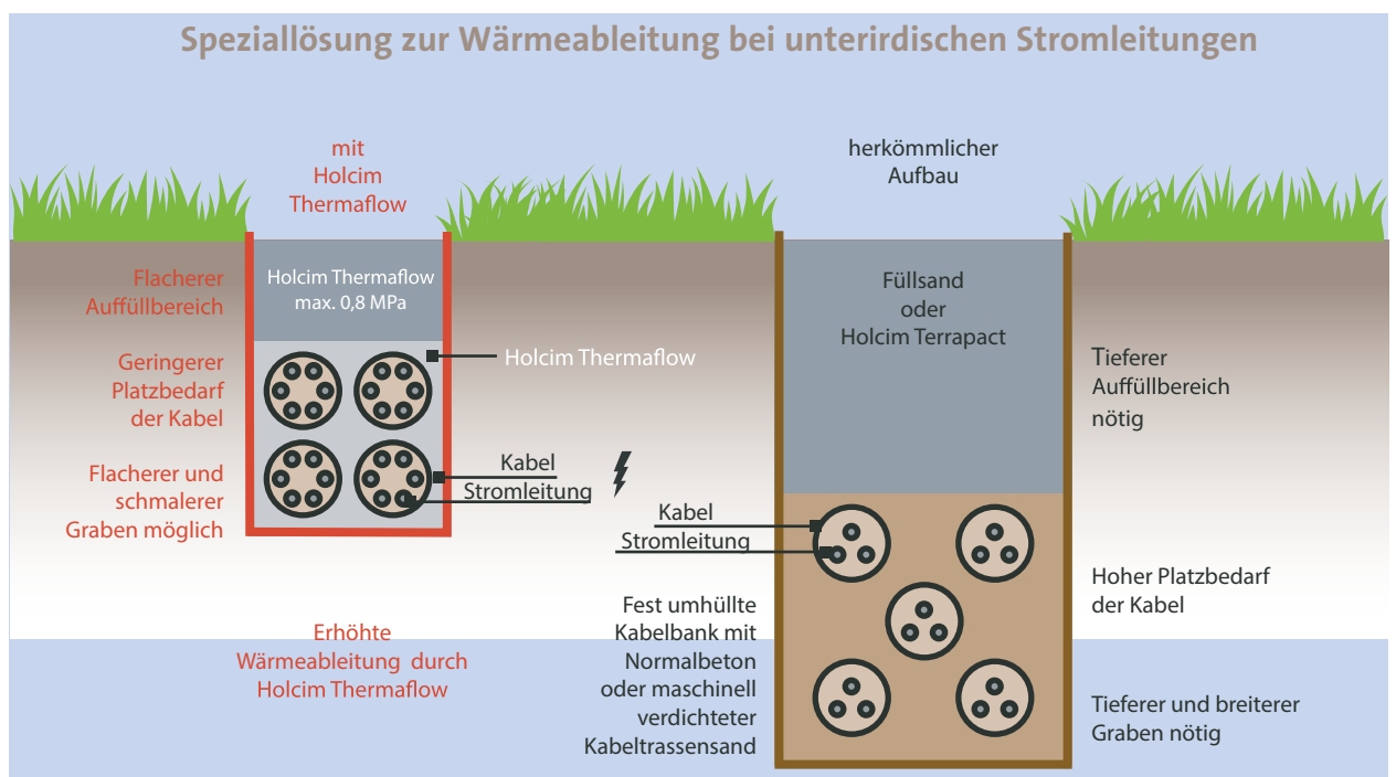
Abb. 7.17.4 Schematische Darstellung von Verfüllungen
