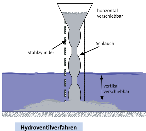
Abb. 8.12.10 (rechts) Pumpverfahren
