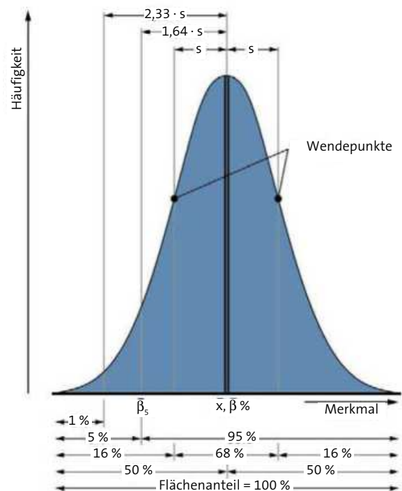
Abb. 6.1.1 Gauß'sche Normalverteilung
