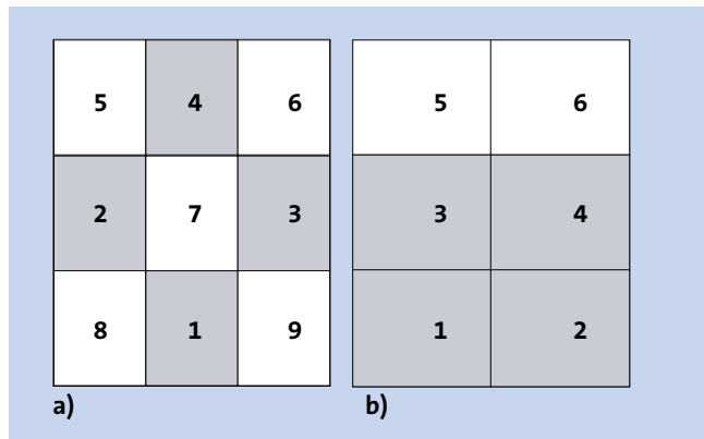
Abb. 10.3.3 Wahl der Betonierabschnitte bei einer Bodenplatte (Grundriss) a) Ungünstige Lösung: erhöhtes Rissrisiko b) Günstige Lösung: geringes Rissrisiko
