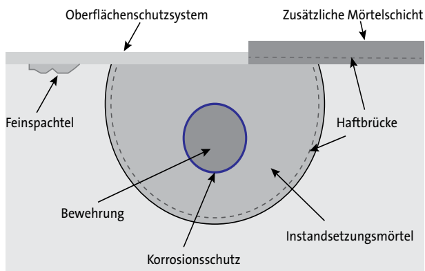
Abb. 8.10.2 Elemente einer Betoninstandsetzung
