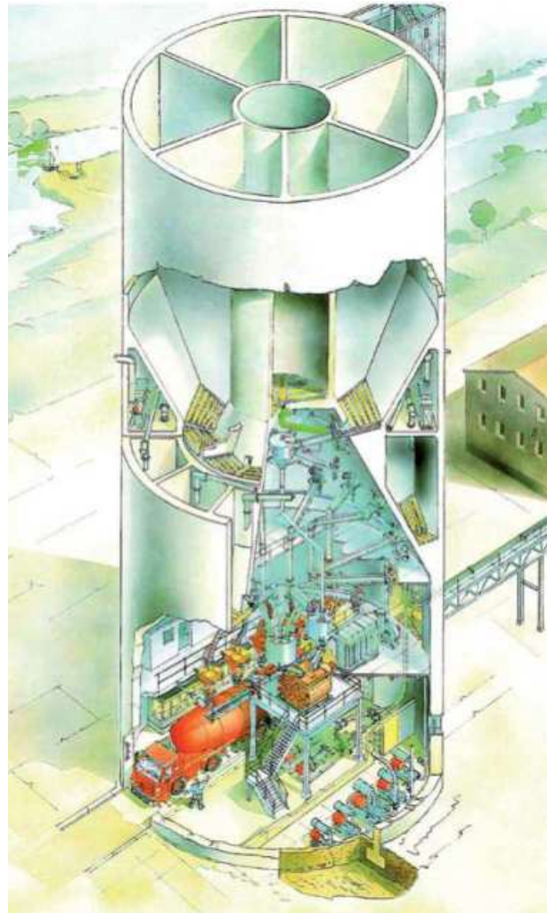
Abb. 1.1.7 Bindemittelmischanlage für Zemente nach Maß
