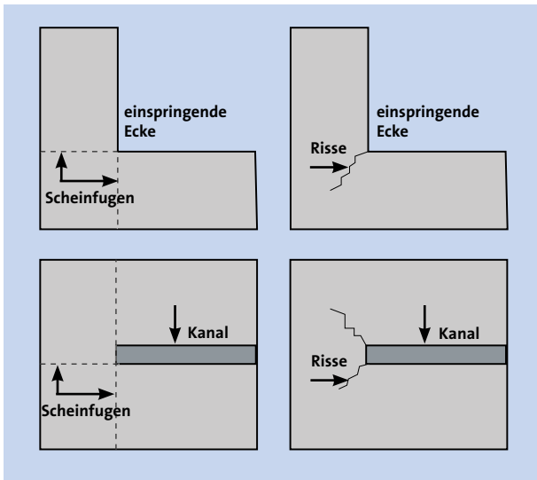
Abb. 8.4.36 Vorschläge der Fugenanordnung bei Stützen, Schächten und Einbauteilen
