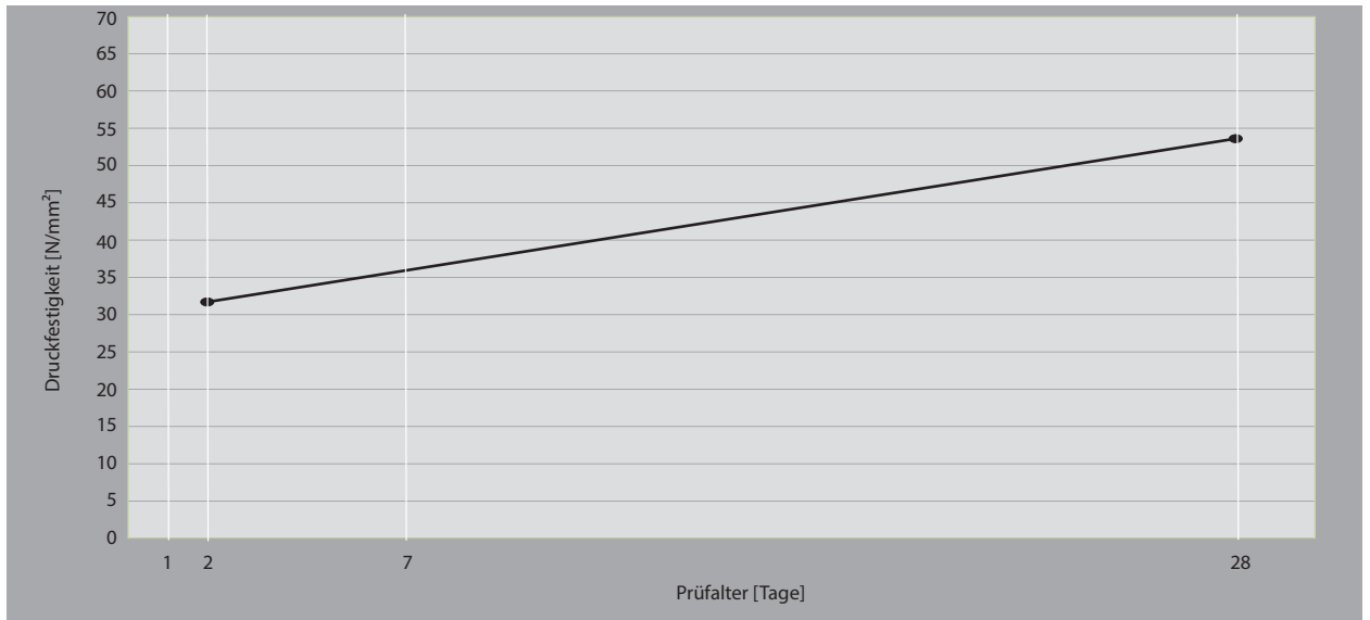
Abb. 5 Druckfestigkeitsentwicklung von Holcim Fluvio 4 N am Normenmörtel nach DIN EN 196
