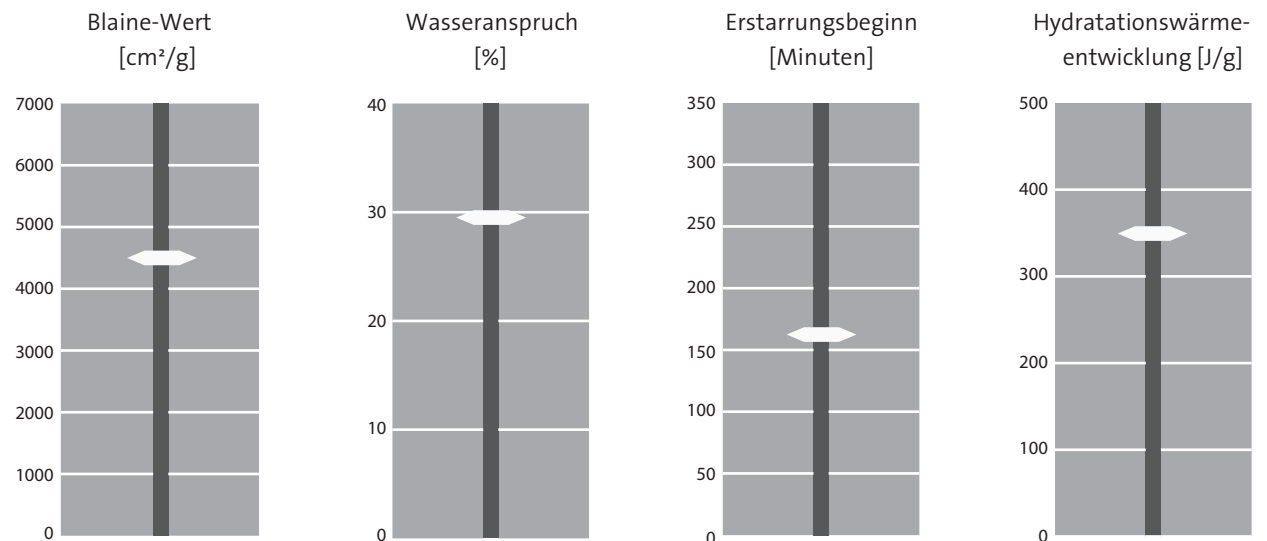
Abb. 6 Technische Daten von Holcim Fluvio 4 N Blaine-Wert, Wasseranspruch, Erstarrungsbeginn und Hydratationswärmeentwicklung
