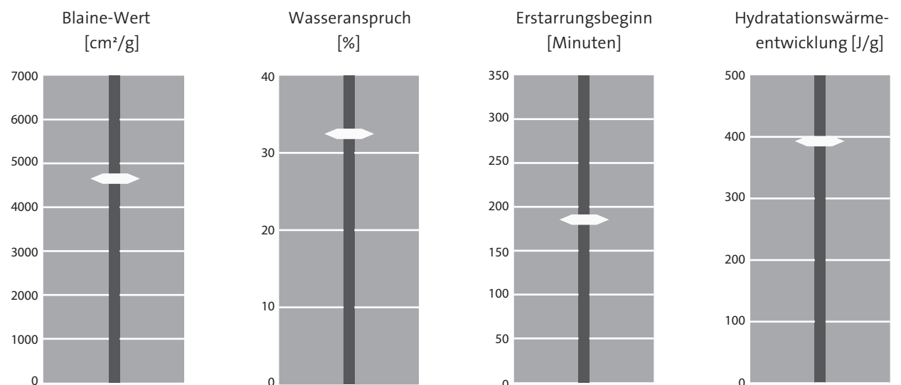
Abb. 6 Technische Daten von Holcim Pur 5 N Blaine-Wert, Wasseranspruch, Erstarrungsbeginn und Hydratationswärmeentwicklung
