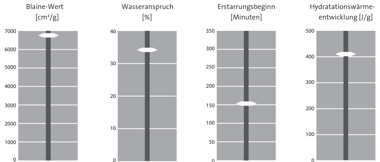
Abb. 6 Technische Daten von Holcim Pur 5 R Blaine-Wert, Wasseranspruch, Erstarrungsbeginn und Hydratationswärmeentwicklung
