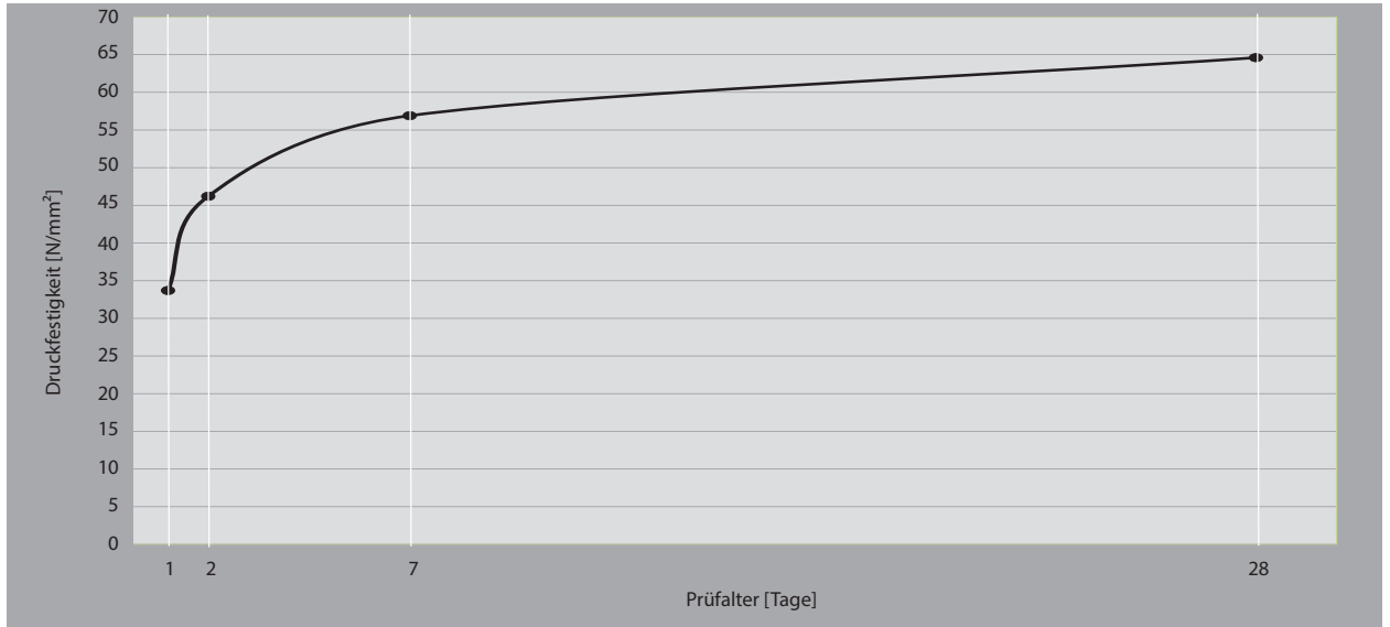
Abb. 5 Druckfestigkeitsentwicklung von Holcim Pur 5 R am Normenmörtel nach DIN EN 196
